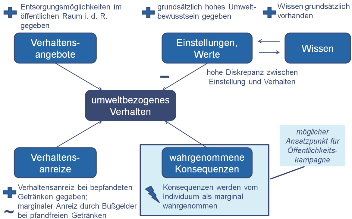
Abbildung 31: Einflussfaktoren auf das Phänomen Littering und Ansatzpunkte für Öffentlichkeitskampagnen
