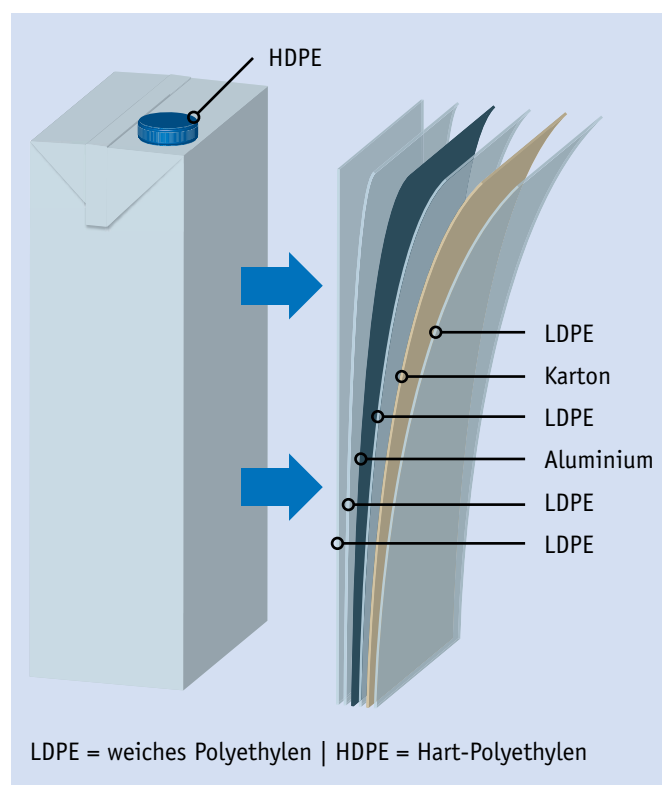
Abbildung 1: Aufbau eines Getränkekartons
