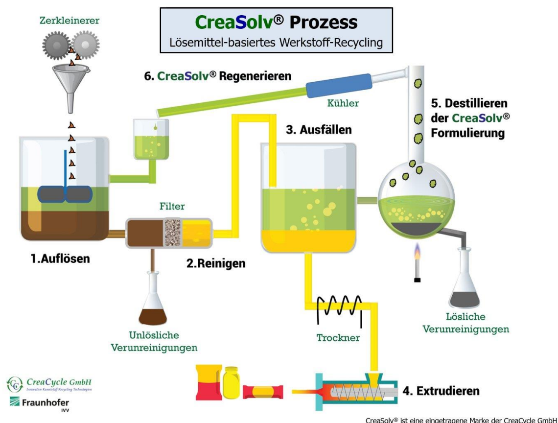
Abbildung 21: Der CreaSolv® Prozess.
