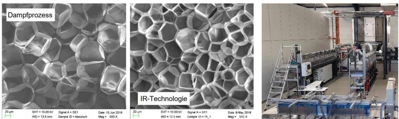
Abbildung 1: Vergleich konventionelles und strahlungsbasiertes Schäumen (links/Mitte) sowie Verarbeitungsanlage der FOX Velution GmbH (rechts)
