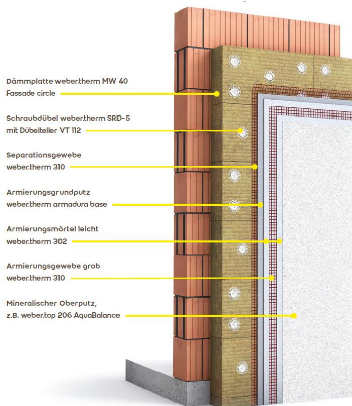
Abbildung 14: Aufbau des recycelbaren WDV-System „Weber.therm circle“. Die Dämmplatte aus Mineralwolle wird mithilfe von Schraubdübeln mit Dübeltellern befestigt. Darauf folgt das Separationsgewebe, welches das sortenreine Trennen der Werkstoffe ermöglicht. Nach dem Armierungsputz, -mörtel und -gewebe folgt der mineralische Oberputz mit AquaBalance-Technologie.
