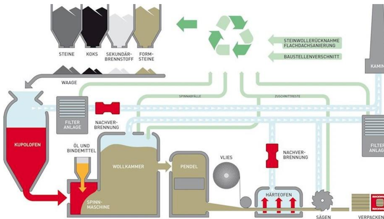
Abbildung 22: Herstellungsprozess Rockwool Steinwolle
