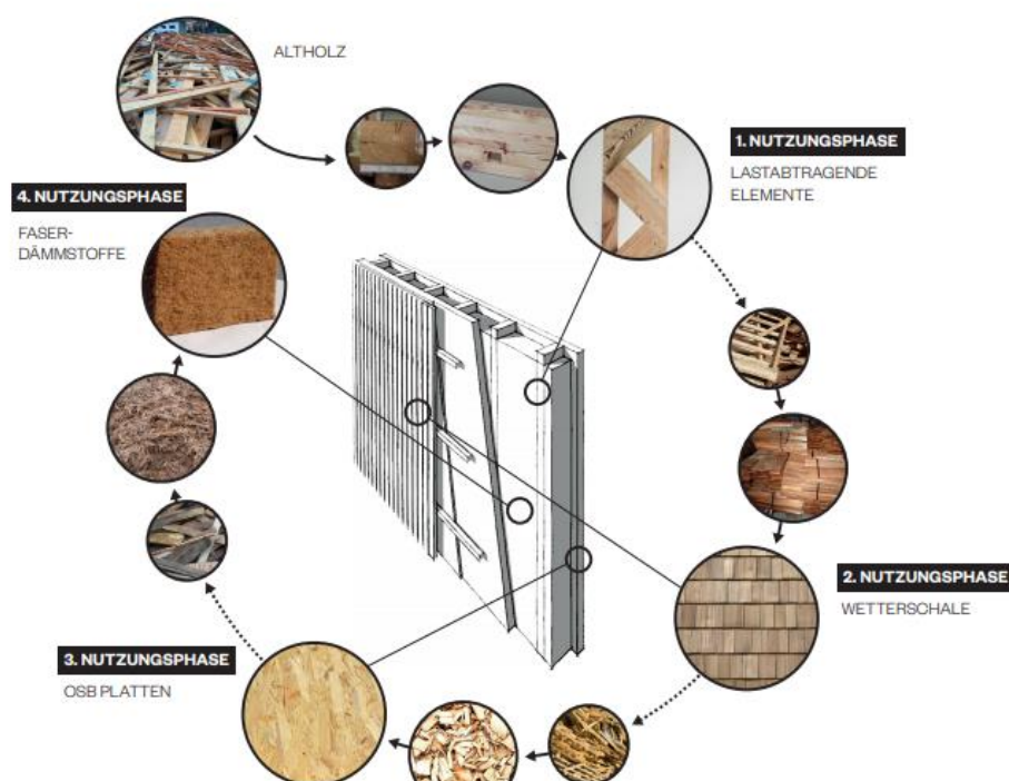
Abbildung 4: Kaskadennutzung von Altholz am Beispiel Fassadenelemente © ZRS Architekten Ingenieure
