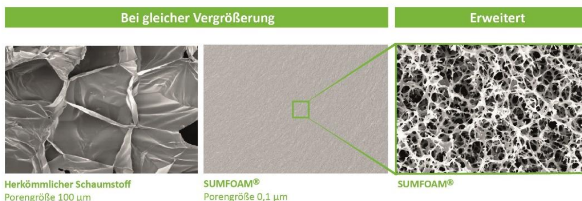
Abbildung 3: SUMFOAM in der Nahansicht
