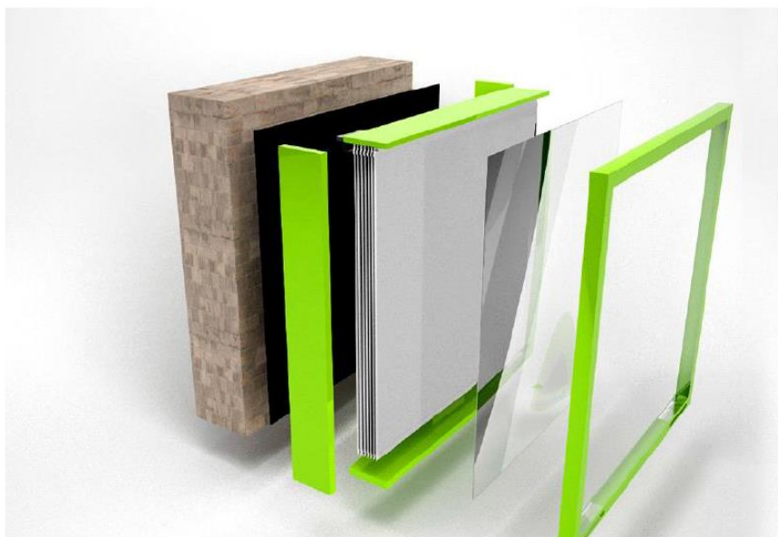
Abbildung 15: 3-D Ansicht der Plusenergiewand. Von hinten nach vorne: Innenwand, absorbierende Farbbeschichtung Rahmen, Folien mit Luftzwischenräumen, Glasabdeckung, Rahmen
