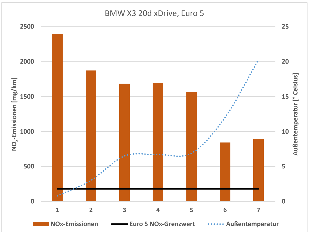
Abb. 3 NO x -Emissionen der einzelnen Messungen
