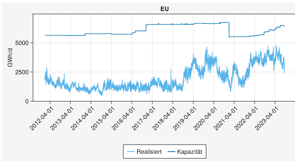
Abbildung 9: Entwicklung der Europäischen LNG-Importe.
