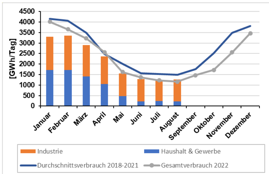
Abbildung 4: Gasverbrauch von Industrie, Haushalten und Gewerbe in Deutschland 2023 im Vergleich zu 2022 und den Jahren 2018-2021 [Monatlicher Mittelwert in GWh/Tag].
