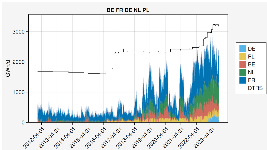
Abbildung 10: Entwicklung der zentraleuropäischen LNG-Importe.
