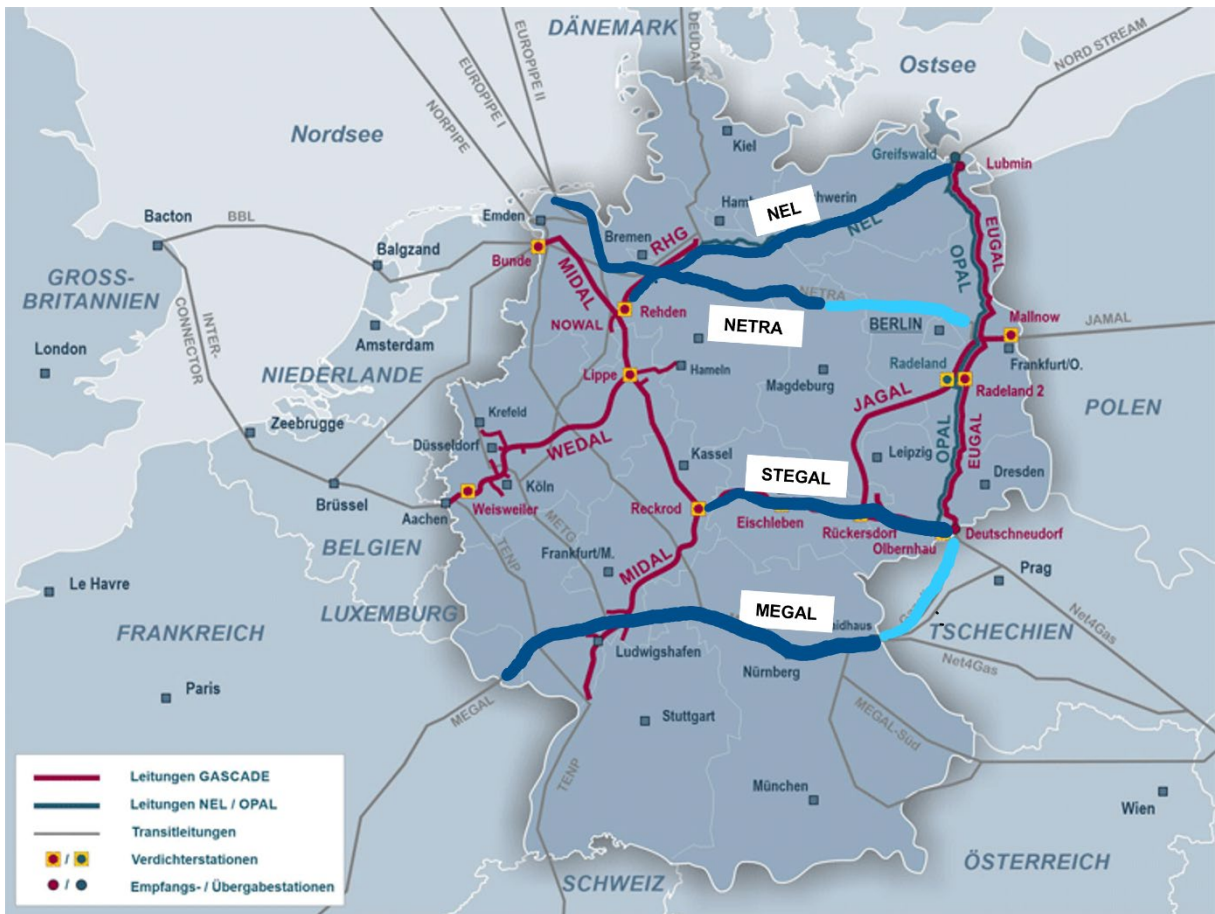
Abbildung 12: Netzkarte Erdgasferntransport in Deutschland.
