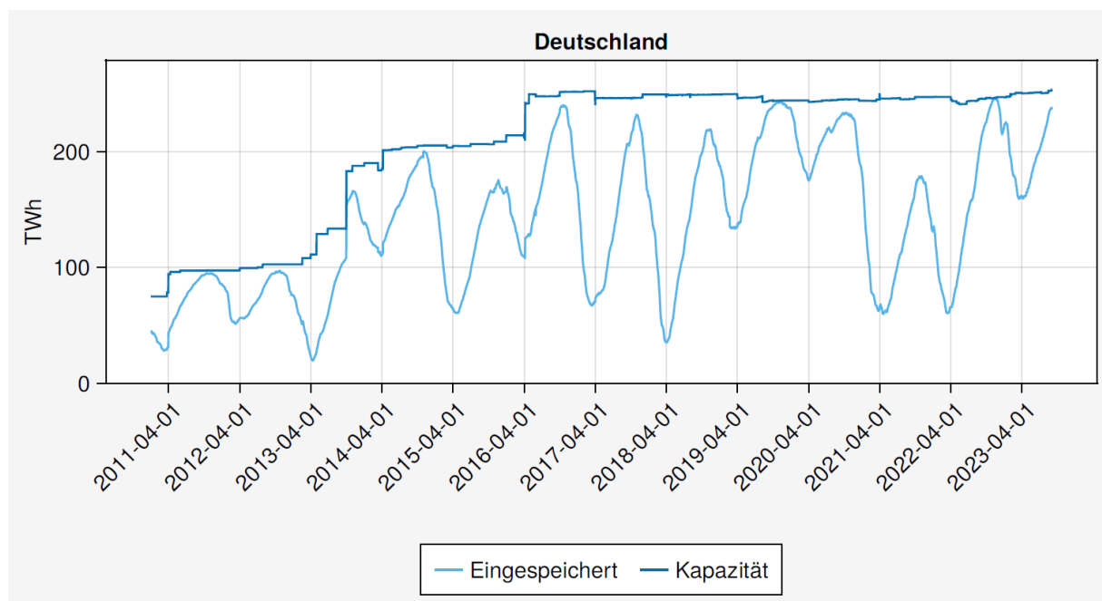
Abbildung 8: Deutsche Speicherfüllstände 2011 – 2023 [TWh].
